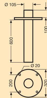
Maße in mm Erdrohr: Art. 3001 zu Kandelaber Art. 3023
